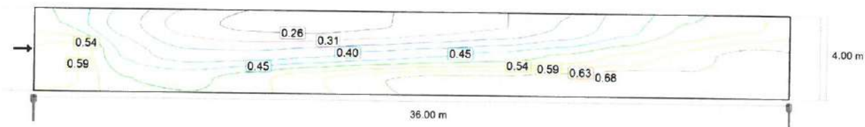
Observator 1: Densitatea luminii la instalația nouă [cd/m 2 ] (Linii Isolux)
