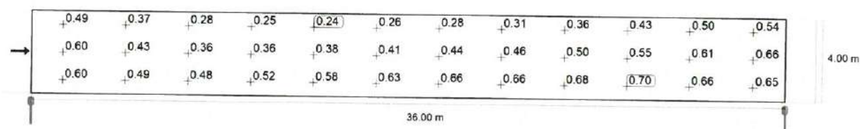
Observator 1: Densitatea luminii la instalația nouă [cd/m 2 ] (Raster valoric)
