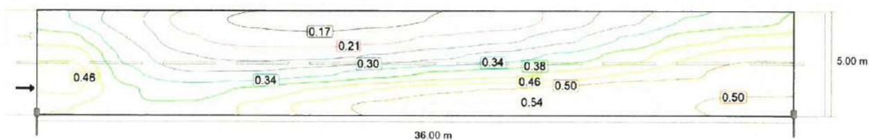
Observator 1: Valoarea de întreținere, densitatea luminii cu carosabil uscat [cd/m 2 ] (Linii Isoluș)
